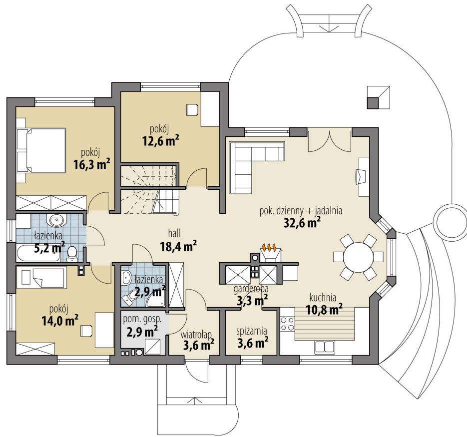
RZUT PARTER
