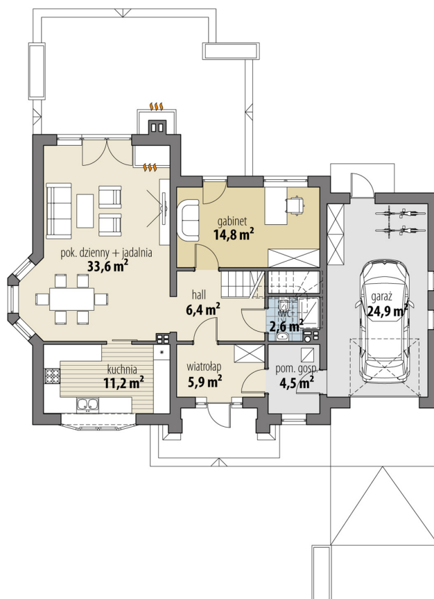
RZUT PARTER
