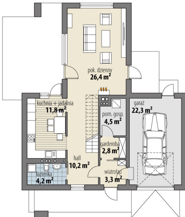
RZUT PARTER
