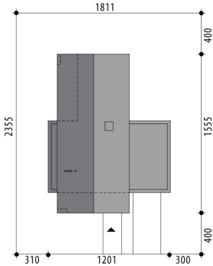
RZUT DZIAŁKI
