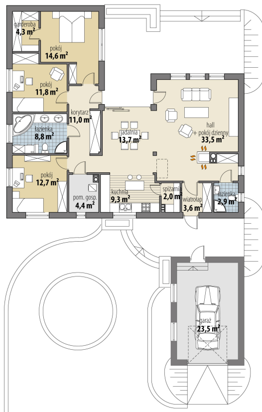
RZUT PARTER
