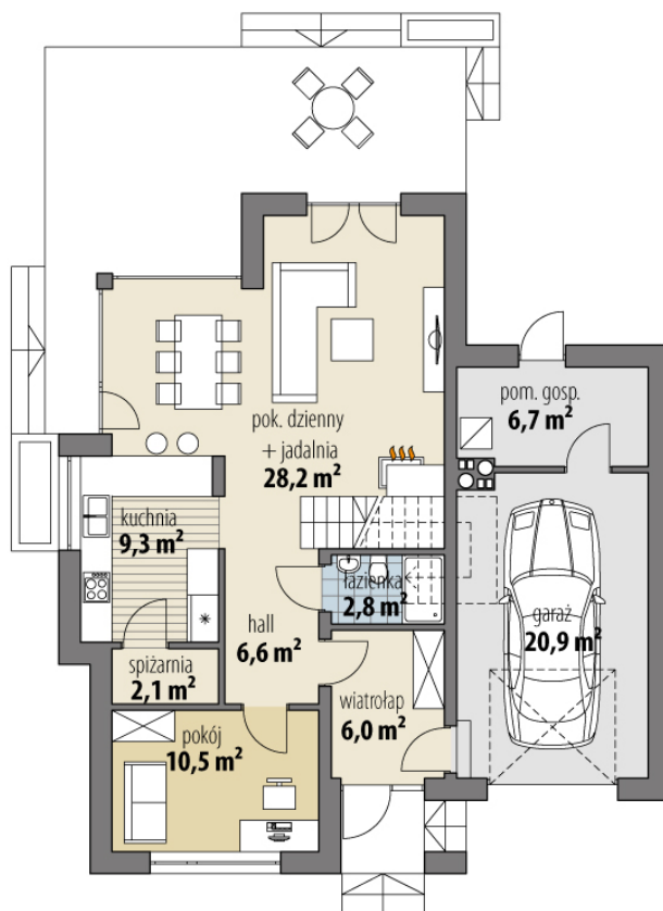
RZUT PARTER
