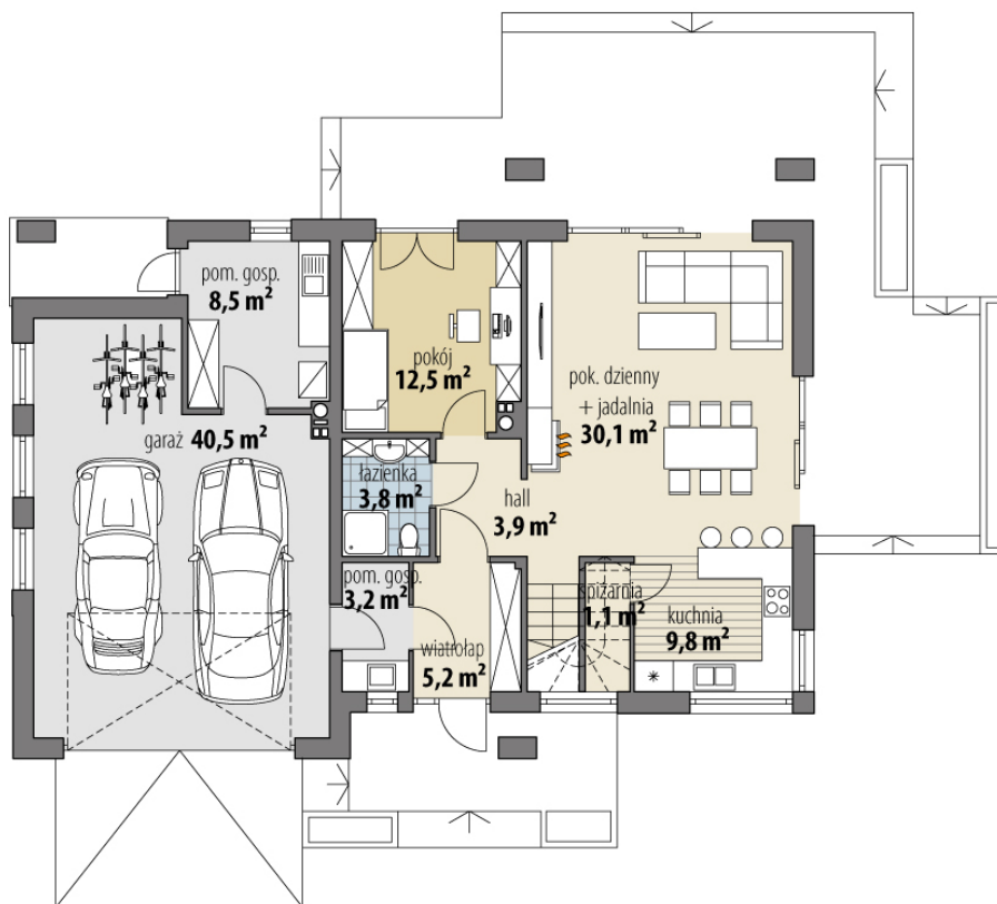
RZUT PARTER
