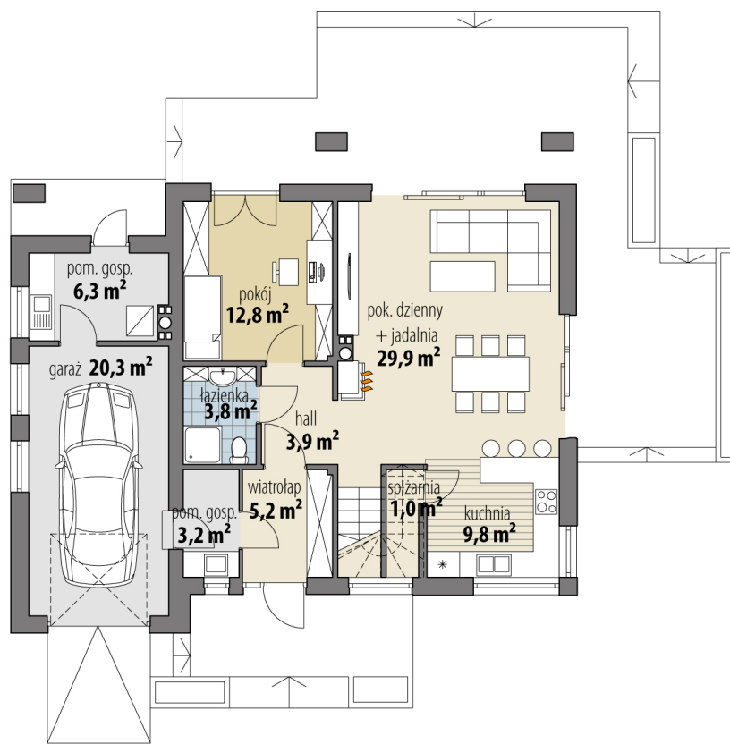
RZUT PARTER
