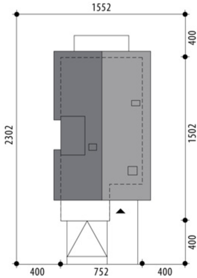
RZUT DZIAŁKI
