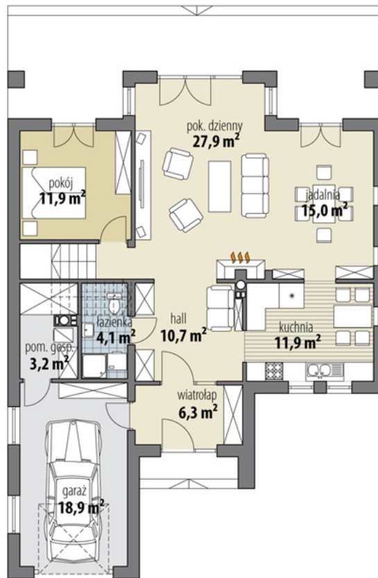
RZUT PARTER
