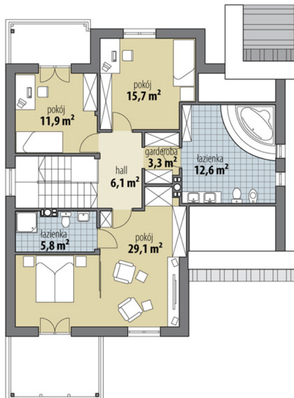
RZUT
