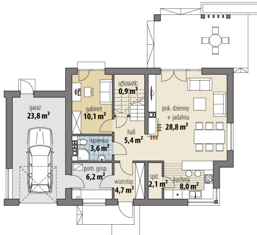
RZUT PARTER
