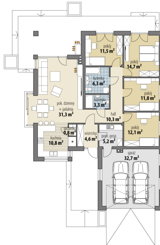
RZUT PARTER
