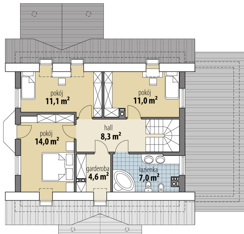
RZUT
