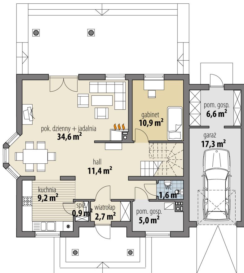
RZUT PARTER
