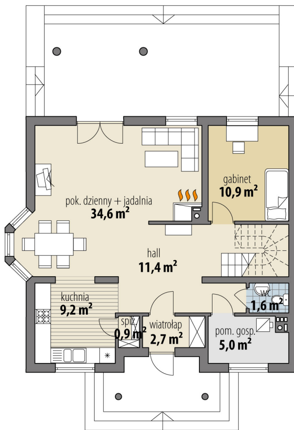
RZUT PARTER
