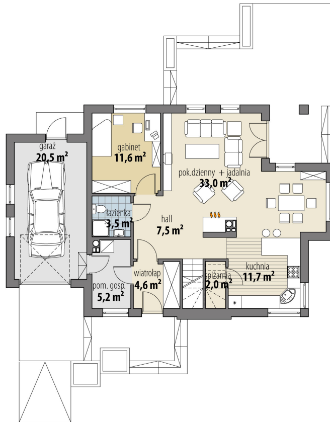
RZUT PARTER
