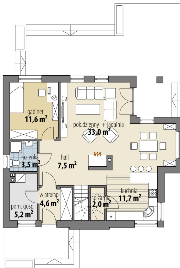
RZUT PARTER
