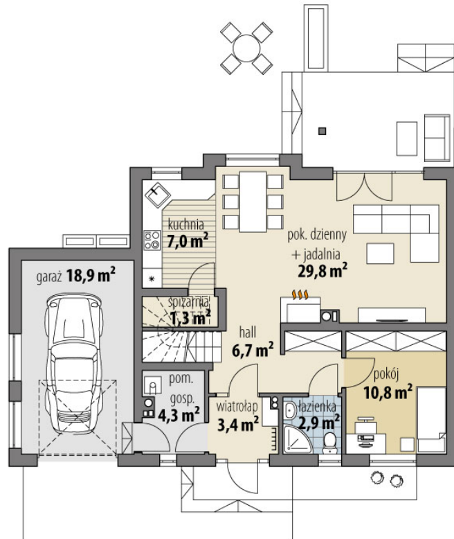
RZUT PARTER
