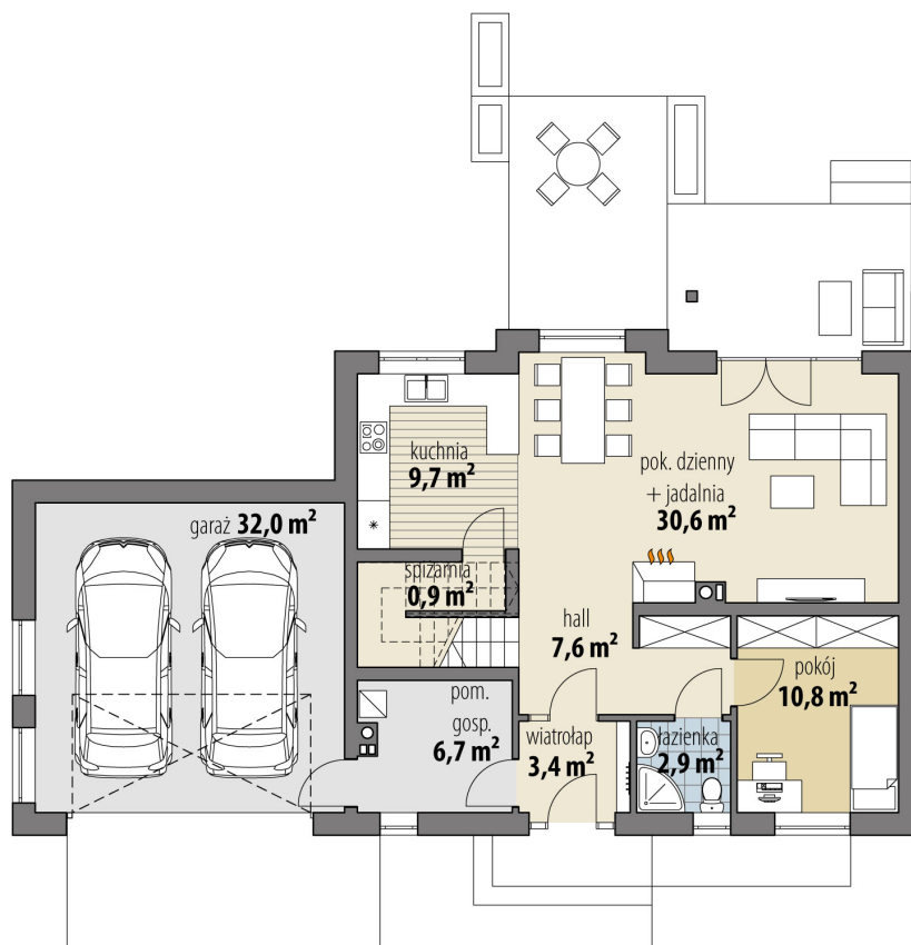
RZUT PARTER
