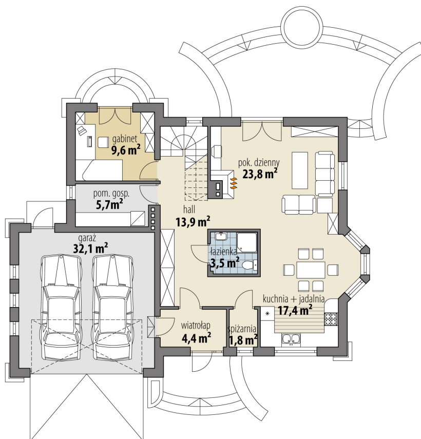
RZUT PARTER
