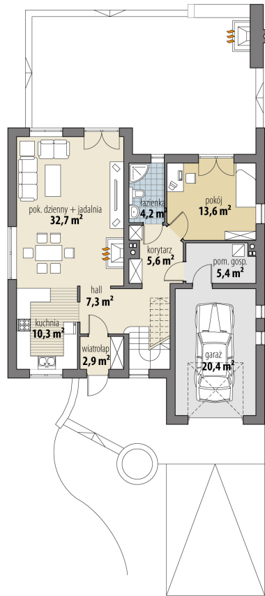
RZUT PARTER
