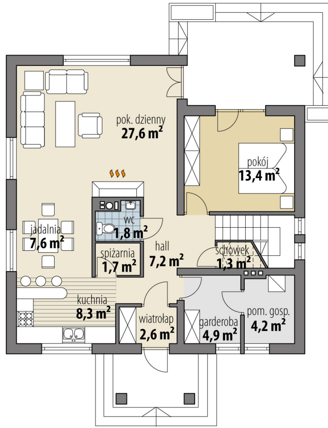
RZUT PARTER
