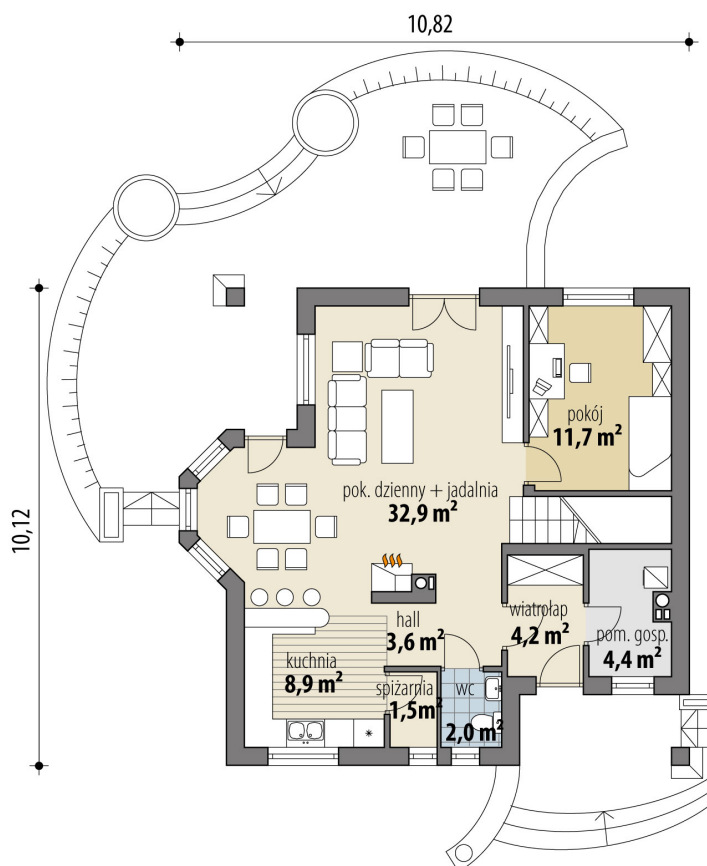
RZUT PARTER
