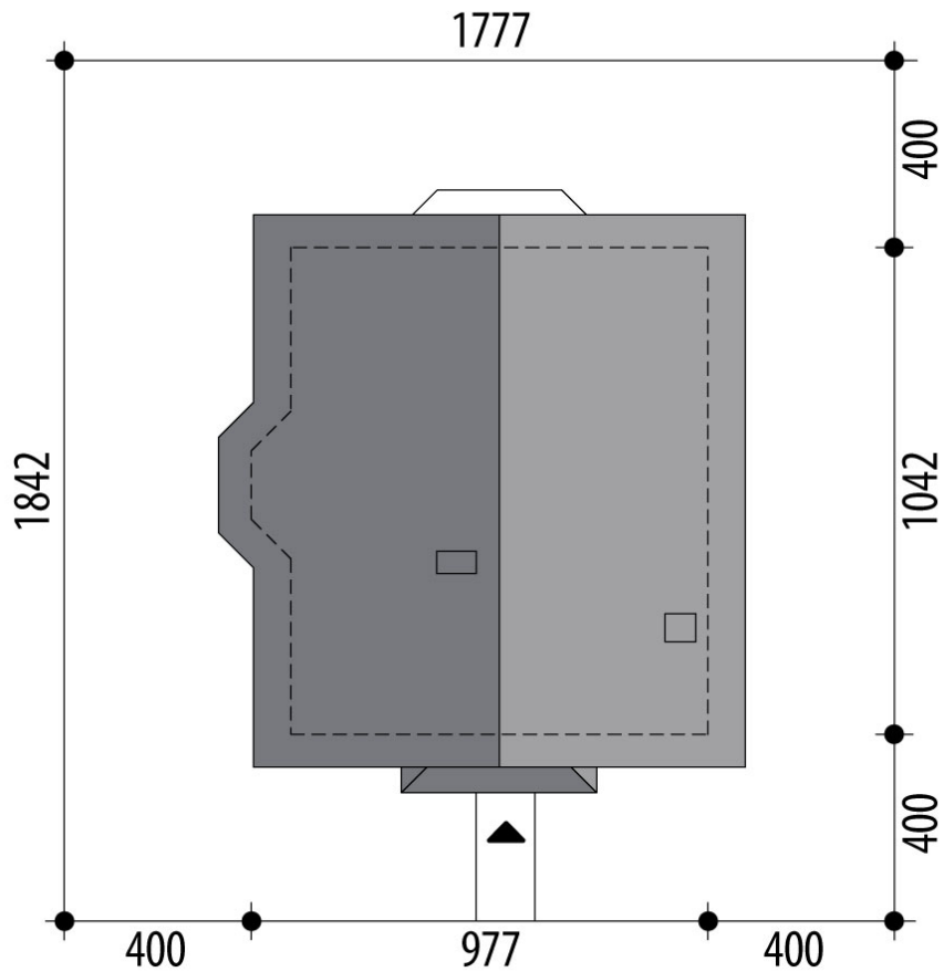
RZUT DZIAŁKI
