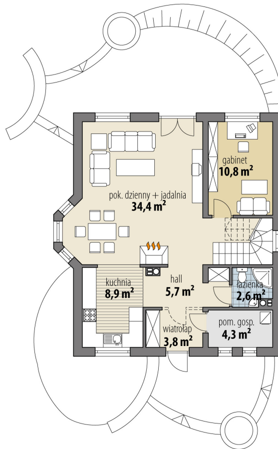
RZUT PARTER
