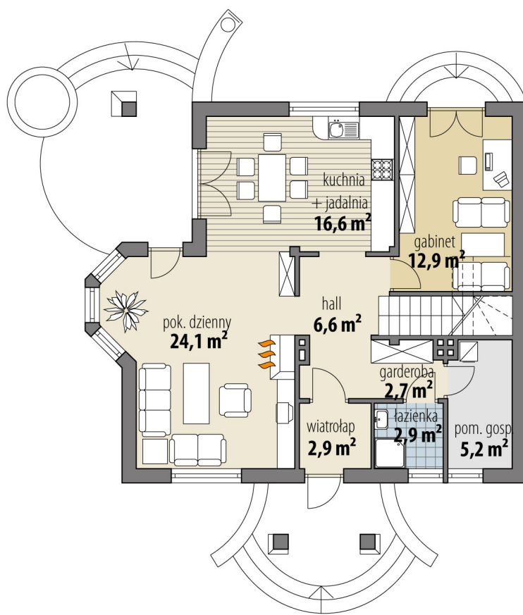
RZUT PARTER
