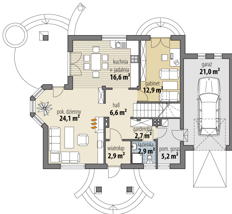
RZUT PARTER
