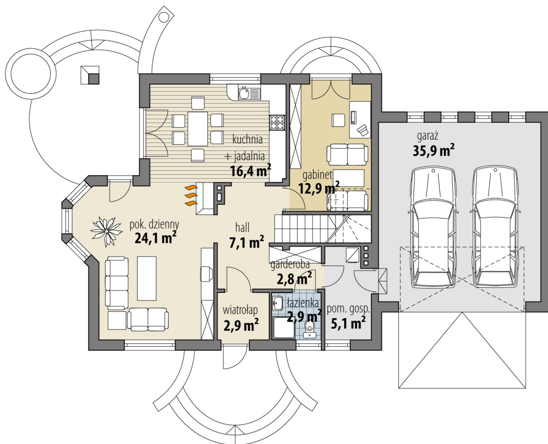
RZUT PARTER
