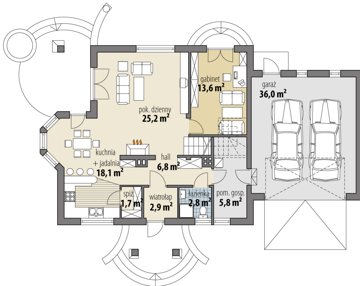
RZUT PARTER
