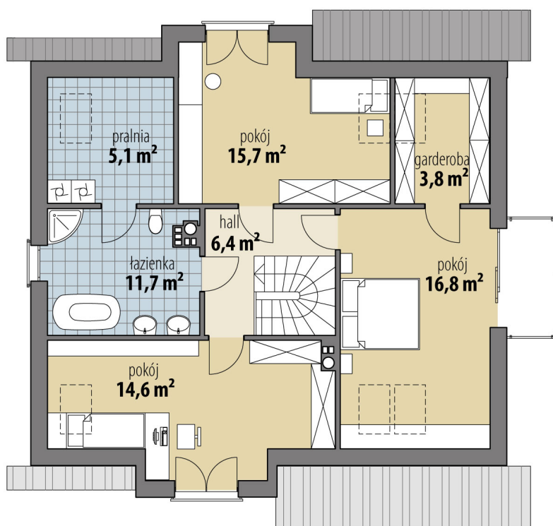
RZUT
