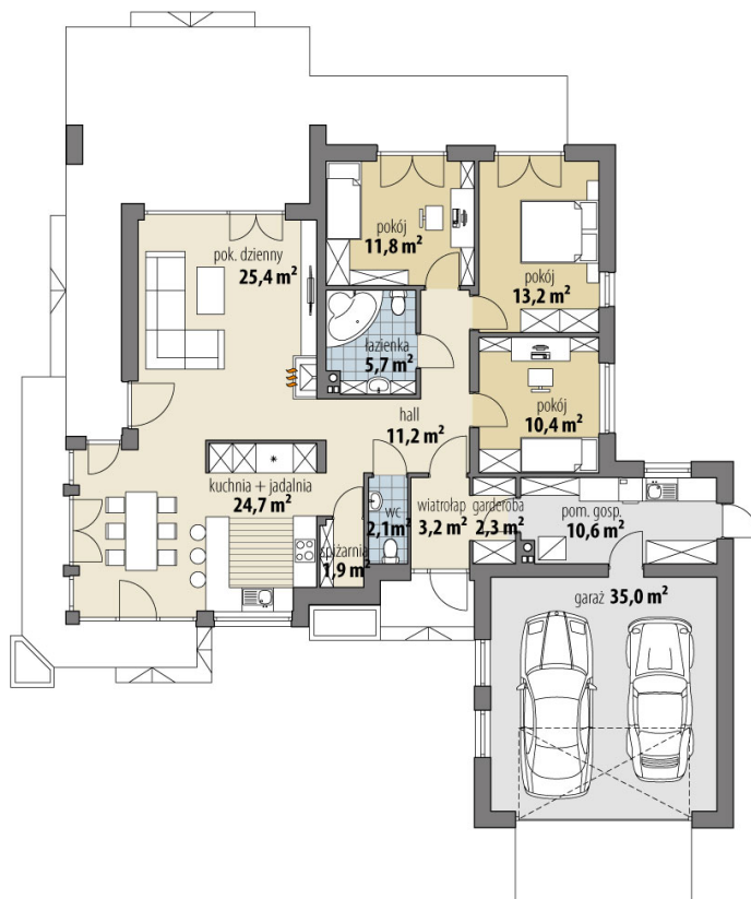
RZUT PARTER
