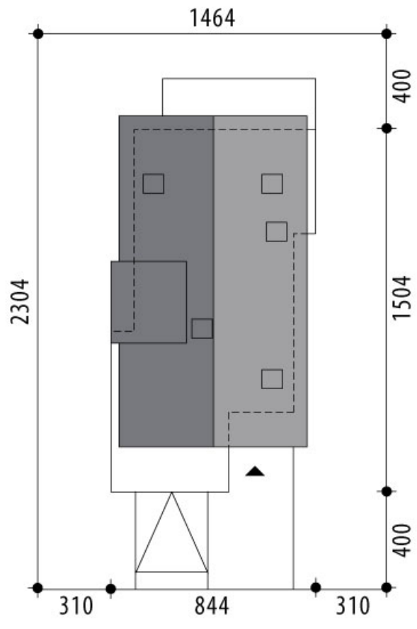
RZUT DZIAŁKI
