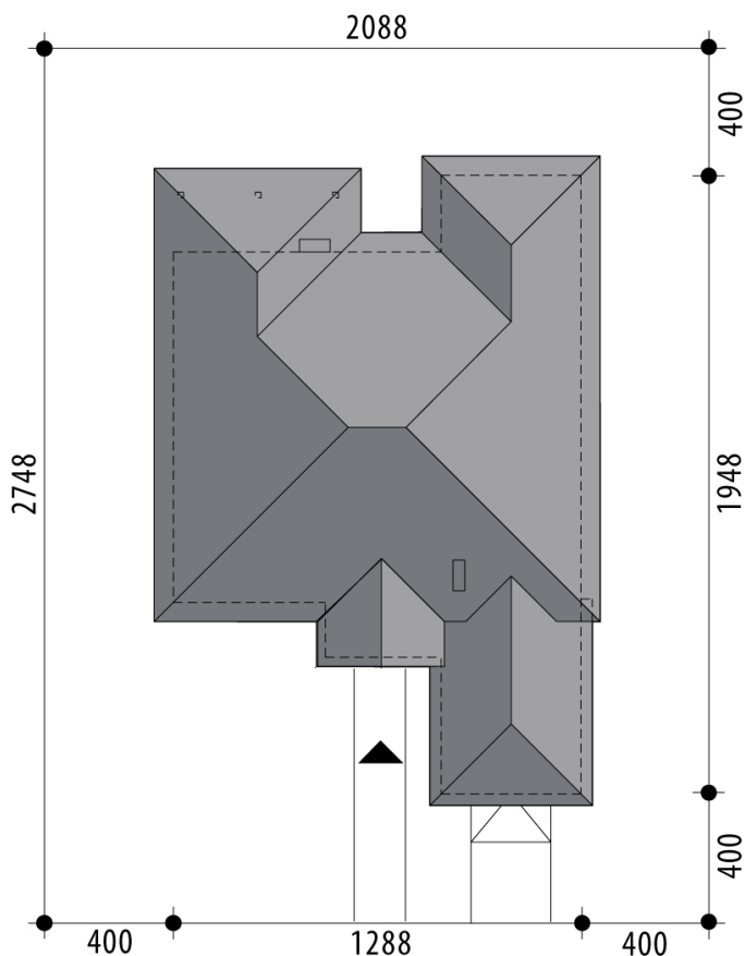
RZUT DZIAŁKI
