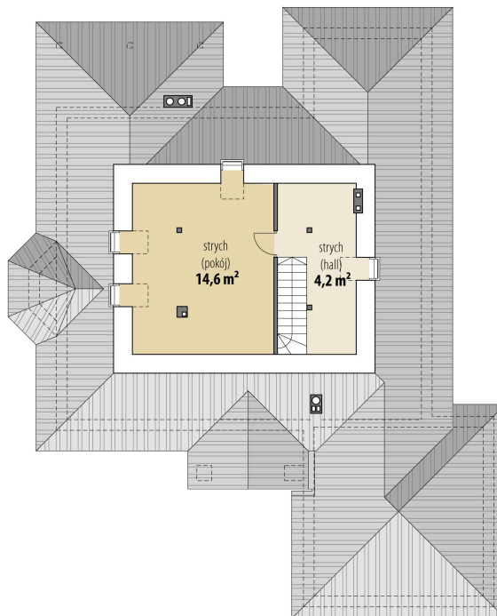
RZUT
