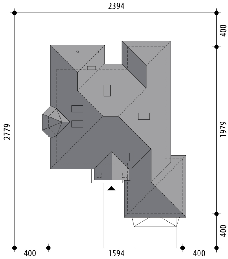
RZUT DZIAŁKI
