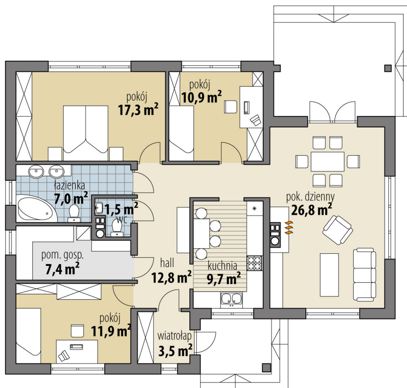
RZUT PARTER
