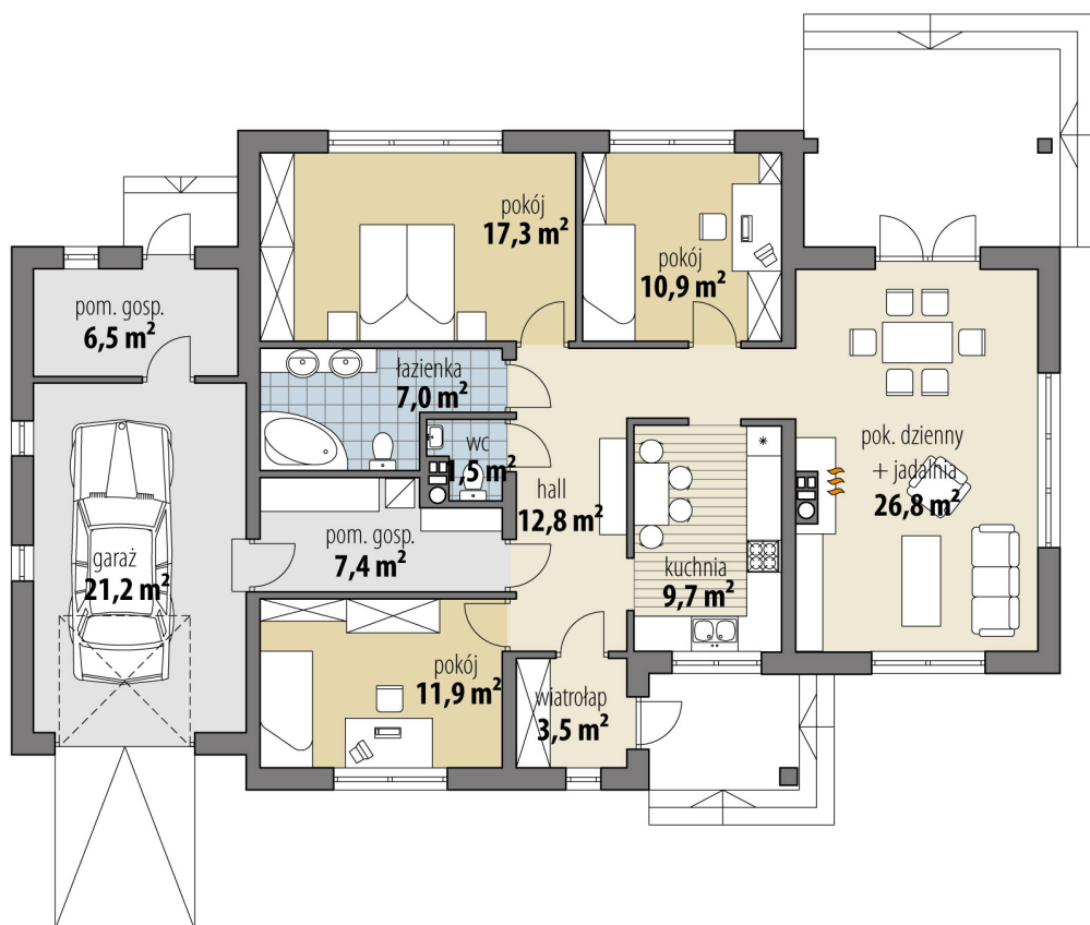
RZUT PARTER
