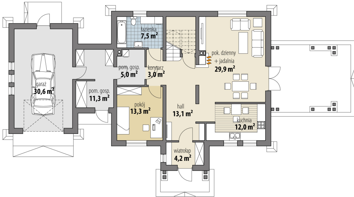
RZUT PARTER
