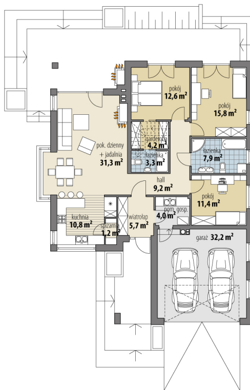
RZUT PARTER
