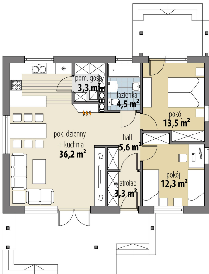
RZUT PARTER
