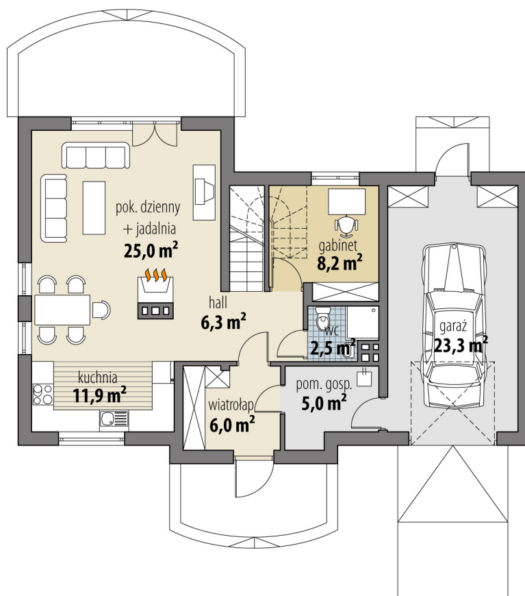
RZUT PARTER
