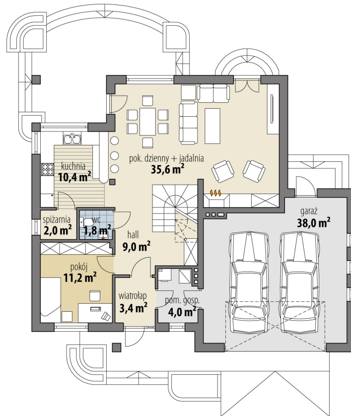
RZUT PARTER
