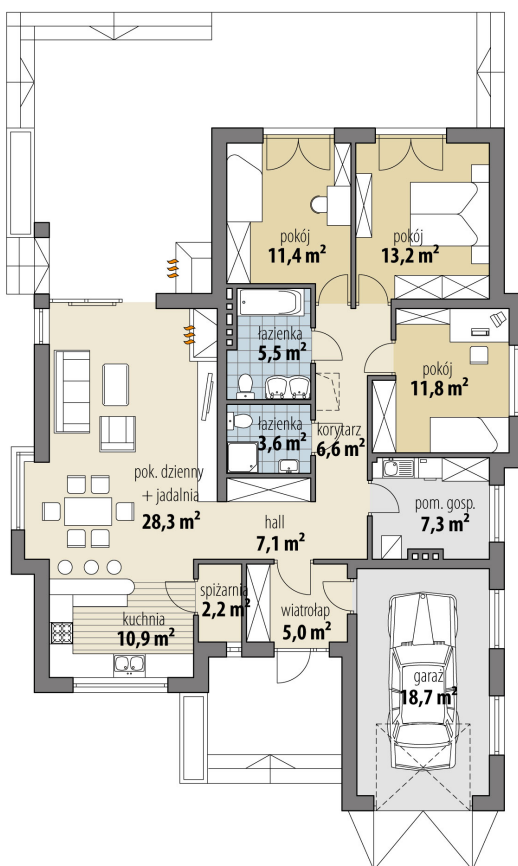
RZUT PARTER
