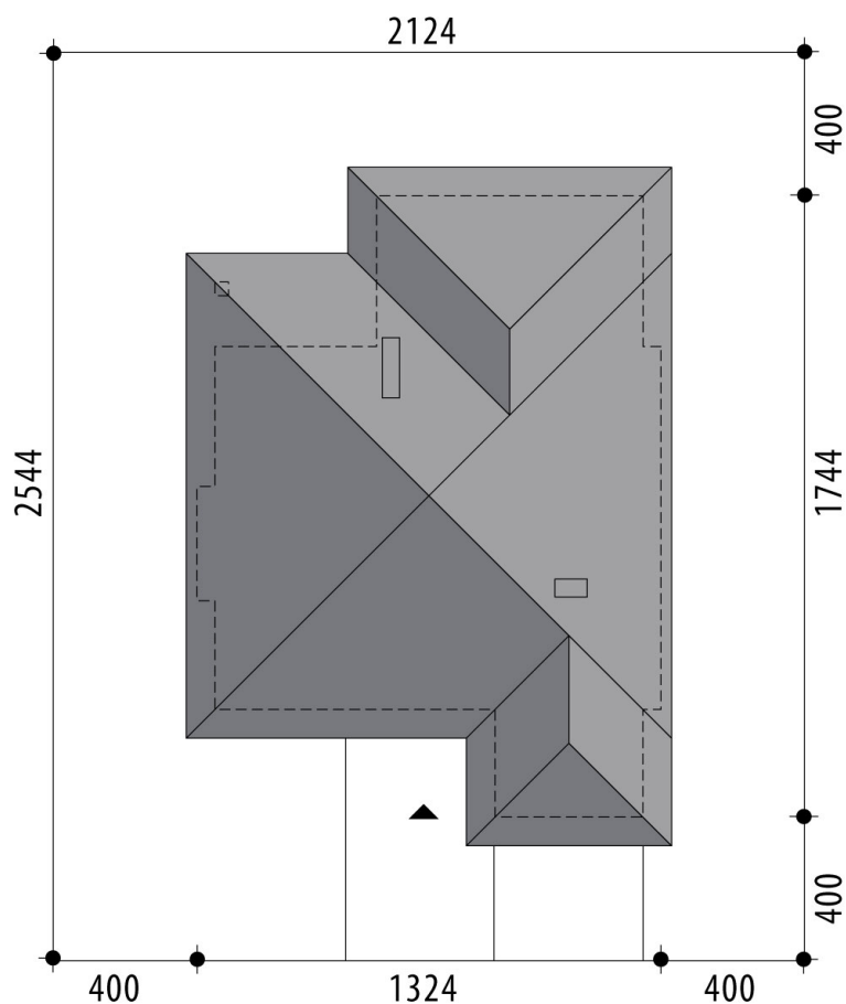
RZUT DZIAŁKI
