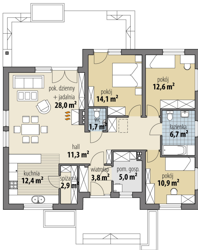
RZUT PARTER
