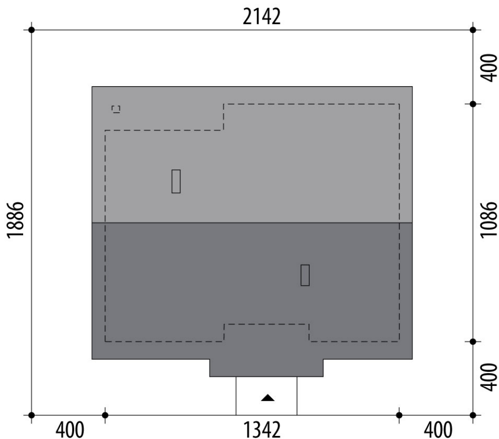
RZUT DZIAŁKI
