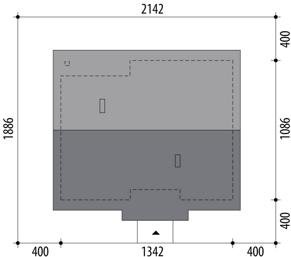
RZUT DZIAŁKI
