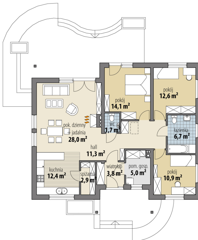
RZUT PARTER
