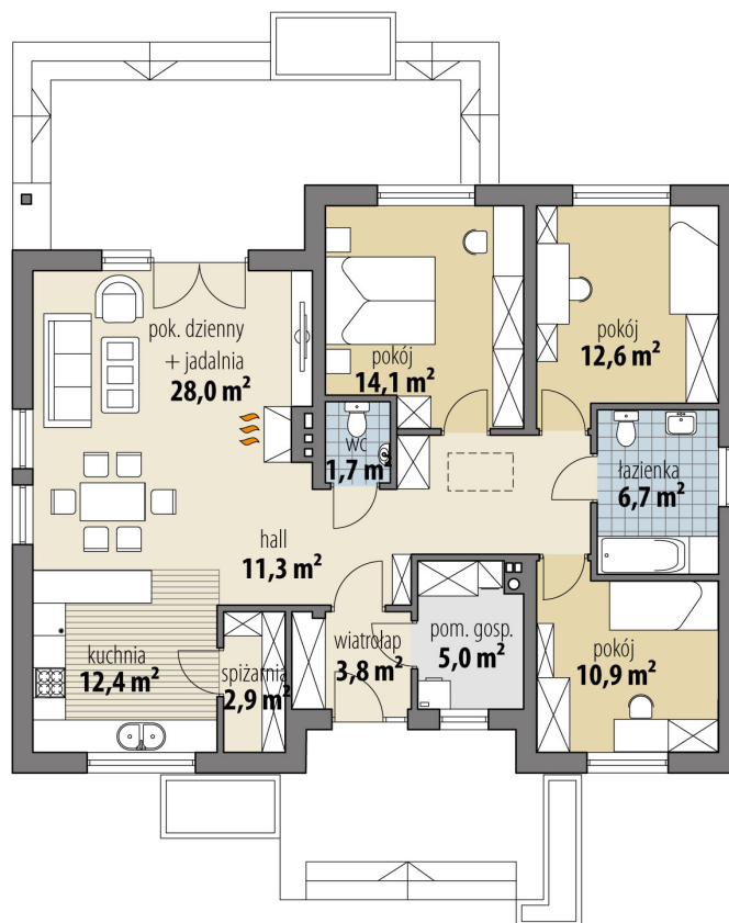
RZUT PARTER
