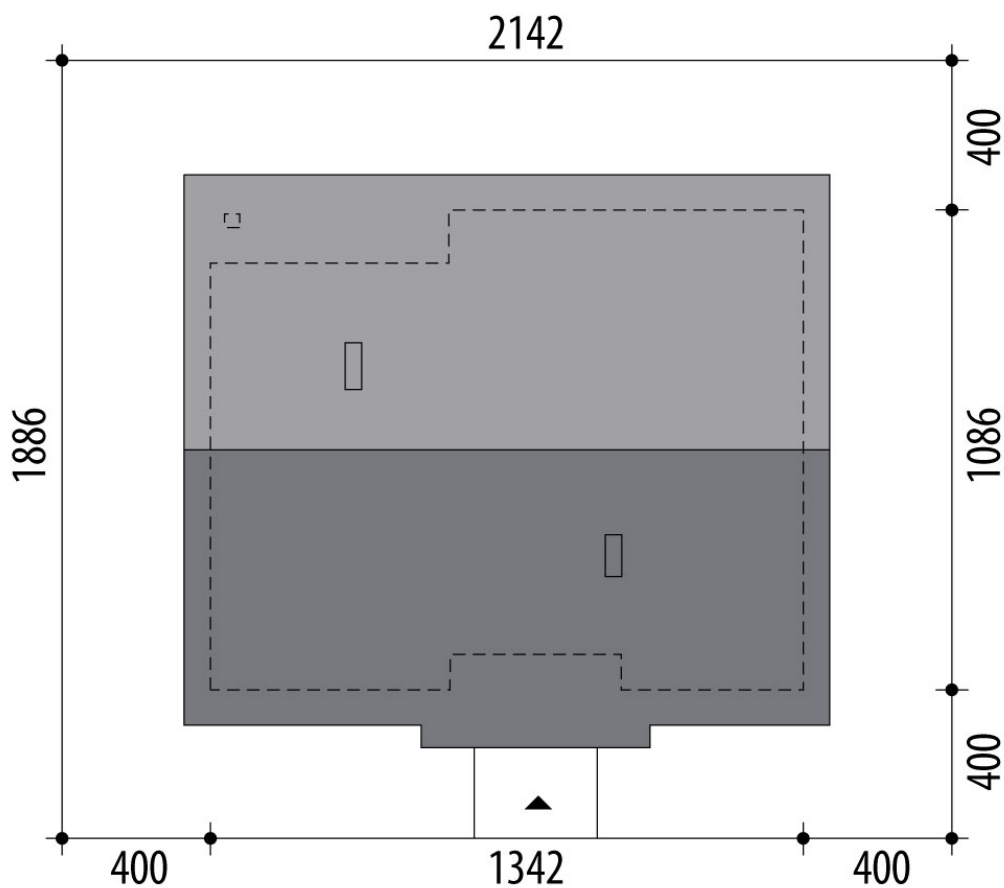
RZUT DZIAŁKI
