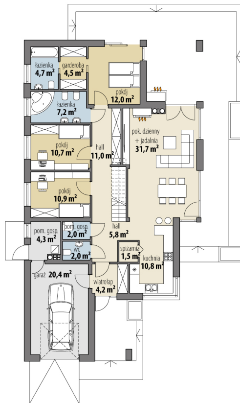
RZUT PARTER
