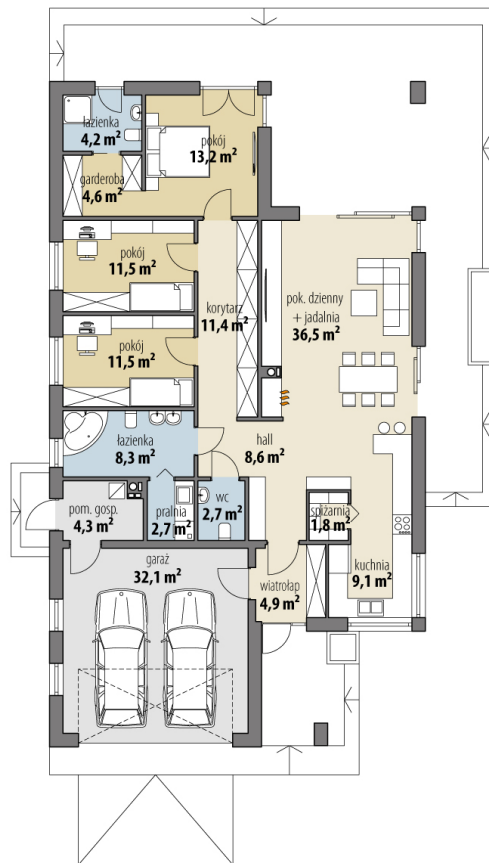
RZUT PARTER
