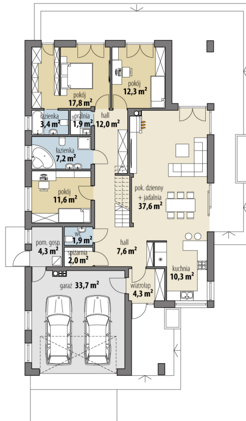
RZUT PARTER
