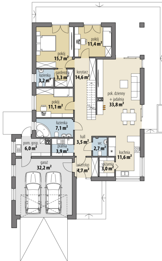
RZUT PARTER
