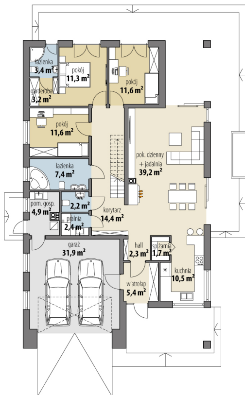
RZUT PARTER
