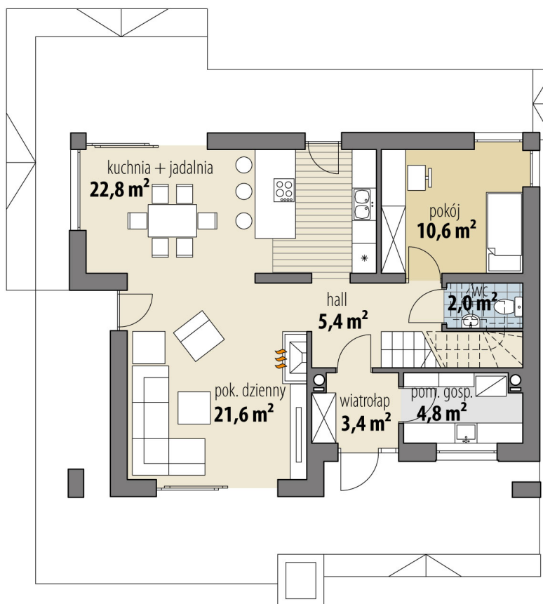
RZUT PARTER
